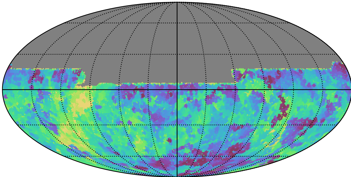
weather_cloudso0v3.5_10yrs All sky u band: Min saturation_mag
