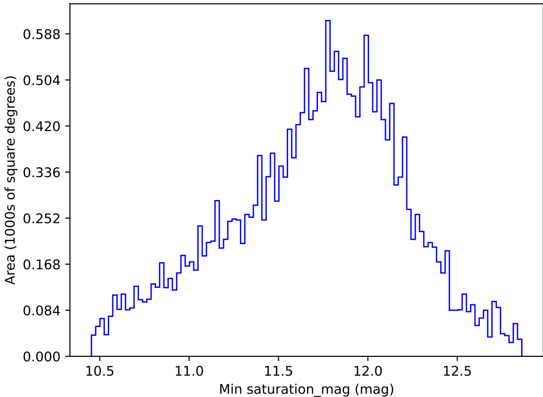
weather_cloudso0v3.5_10yrs All sky u band: Min saturation_mag
