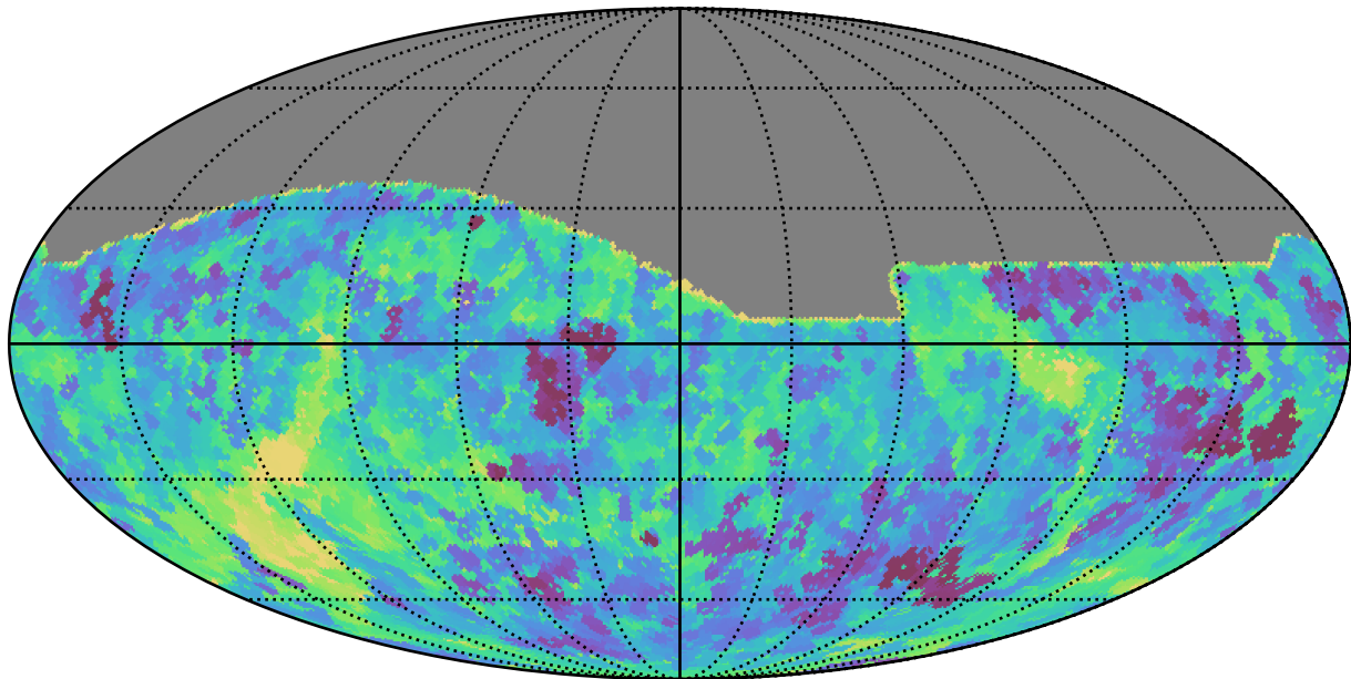
weather_cloudso0v3.5_10yrs All sky r band: Min saturation_mag
