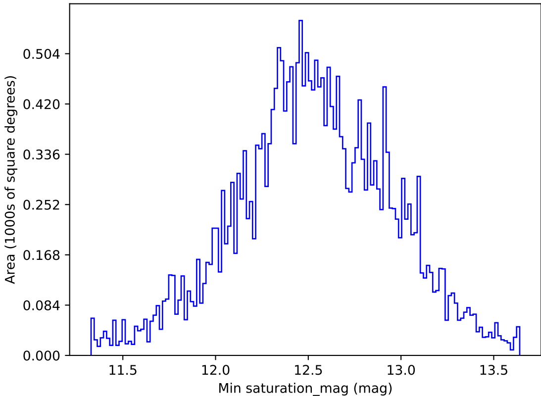
weather_cloudso0v3.5_10yrs All sky r band: Min saturation_mag
