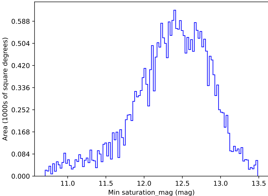
weather_cloudso0v3.5_10yrs All sky i band: Min saturation_mag
