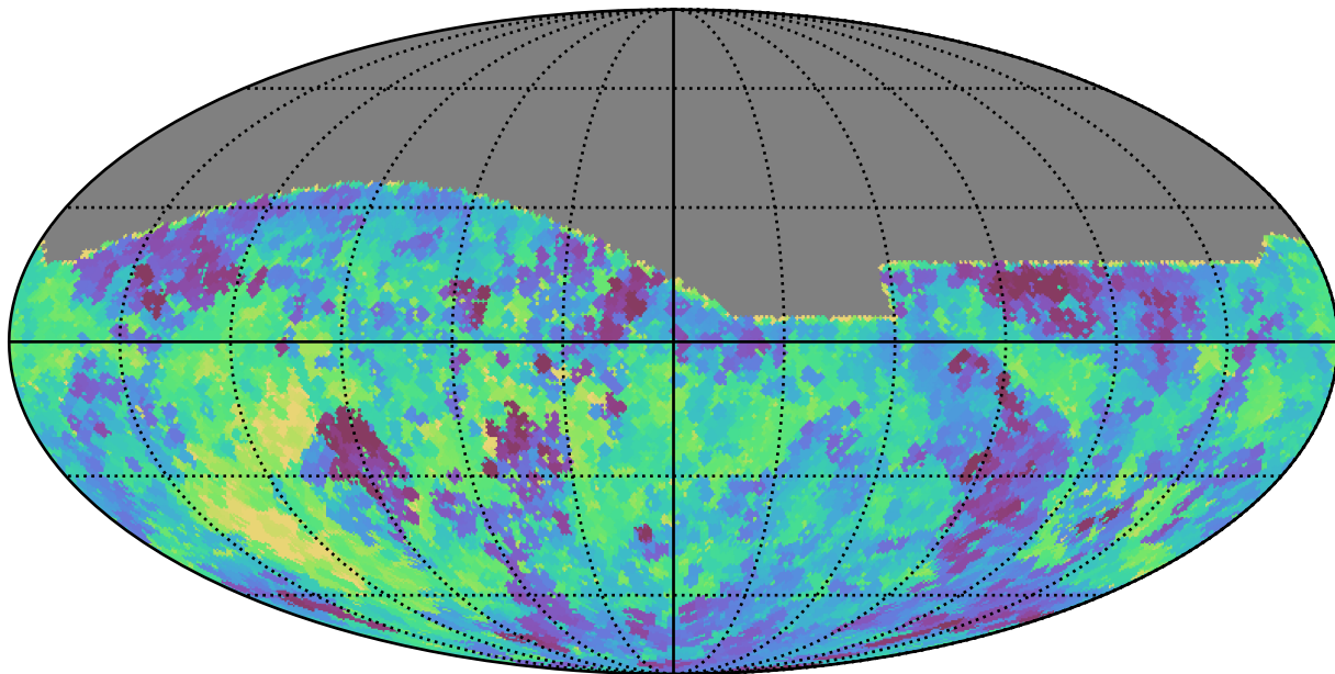
weather_cloudso0v3.5_10yrs All sky g band: Min saturation_mag
