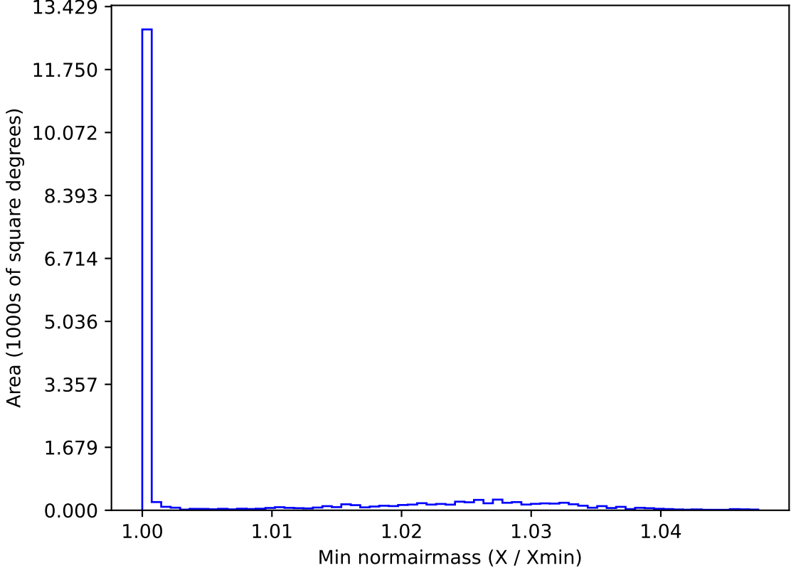
weather_cloudso0v3.5_10yrs WFD y band: Min normairmass
