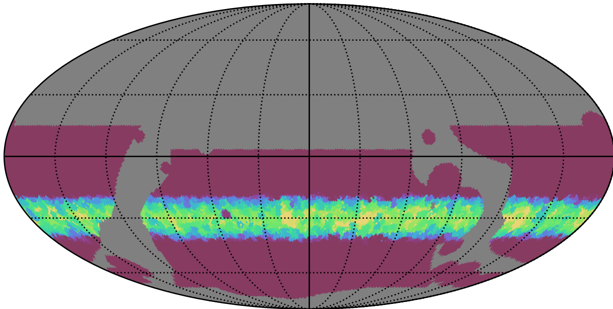
weather_cloudso0v3.5_10yrs WFD i band: Min normairmass
