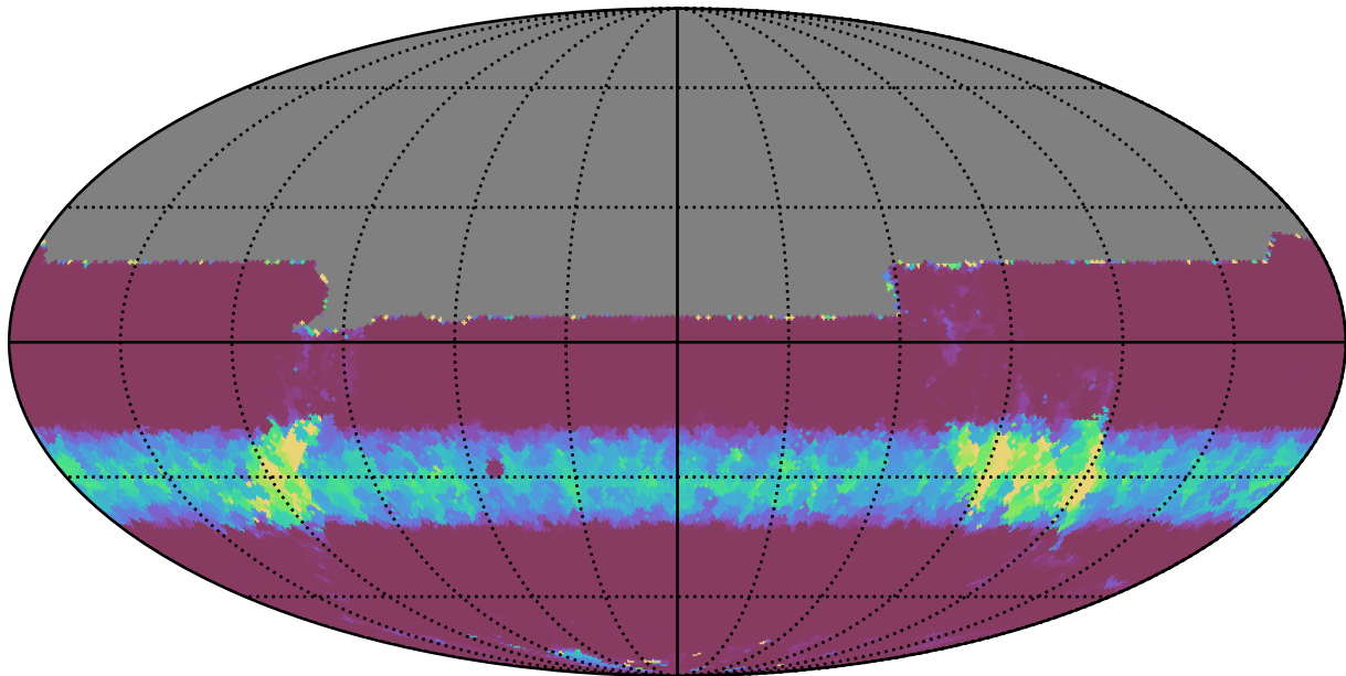
weather_cloudso0v3.5_10yrs All sky y band: Min normairmass
