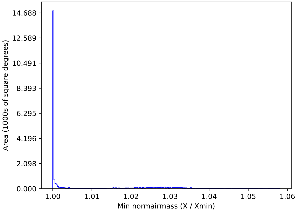
weather_cloudso0v3.5_10yrs All sky y band: Min normairmass
