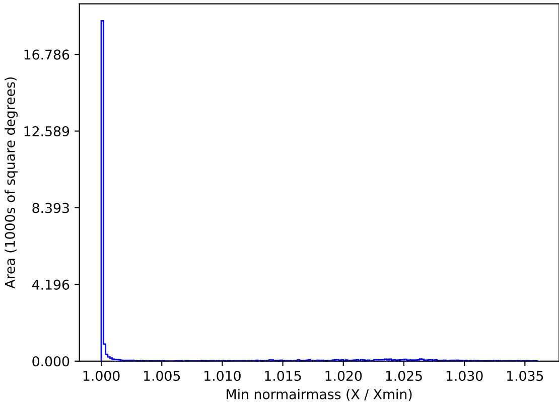
weather_cloudso0v3.5_10yrs All sky i band: Min normairmass
