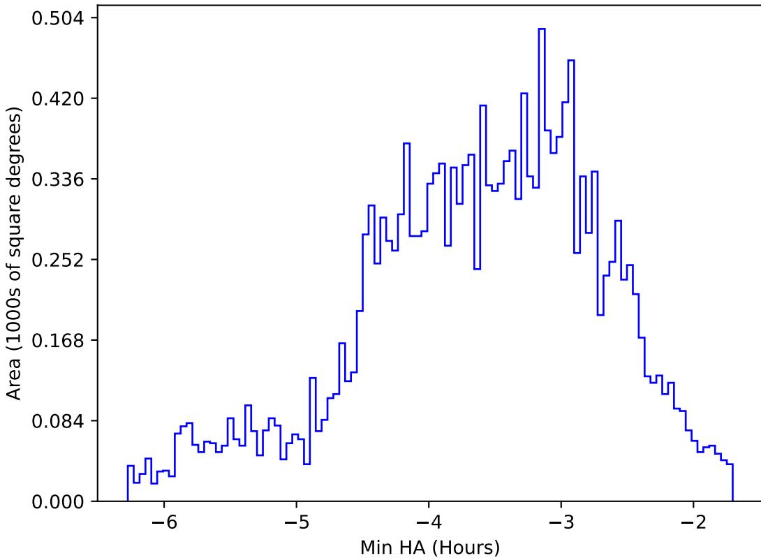
weather_cloudso0v3.5_10yrs WFD y band: Min HA
