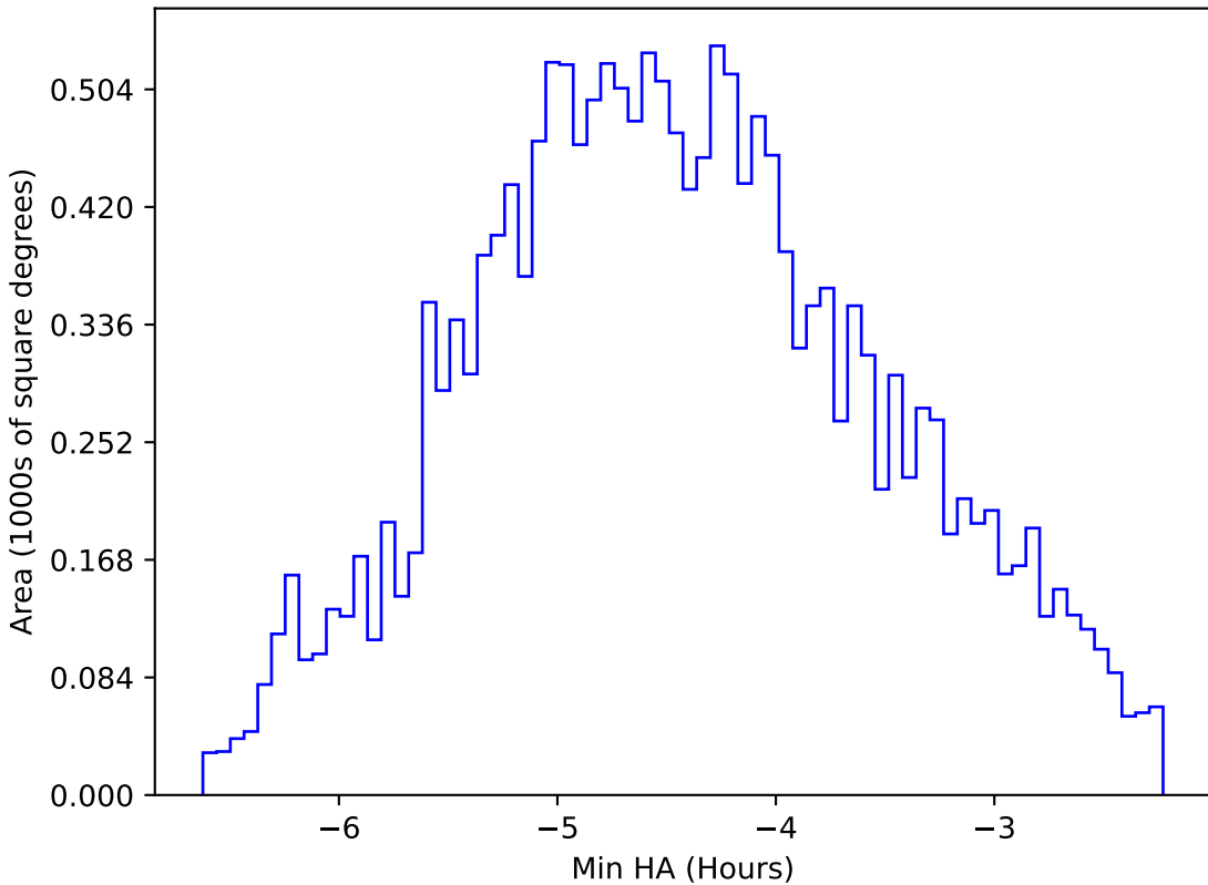
weather_cloudso0v3.5_10yrs WFD i band: Min HA
