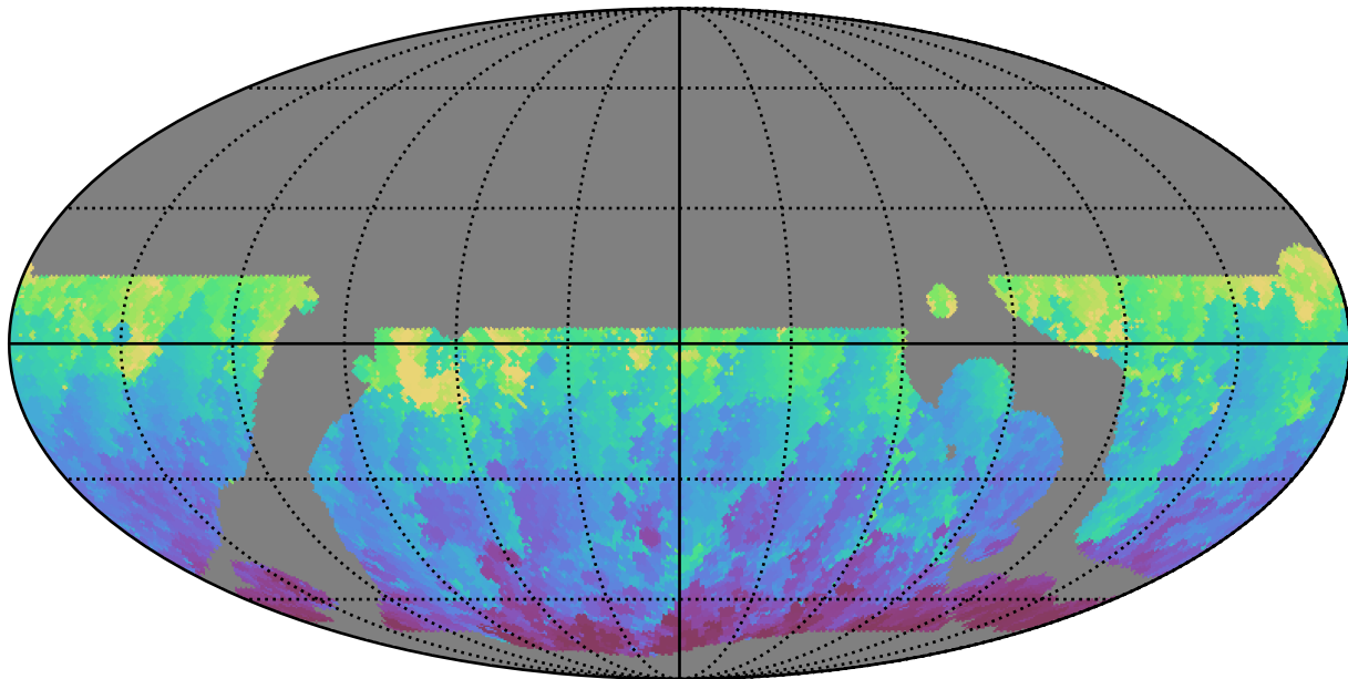
weather_cloudso0v3.5_10yrs WFD g band: Min HA
