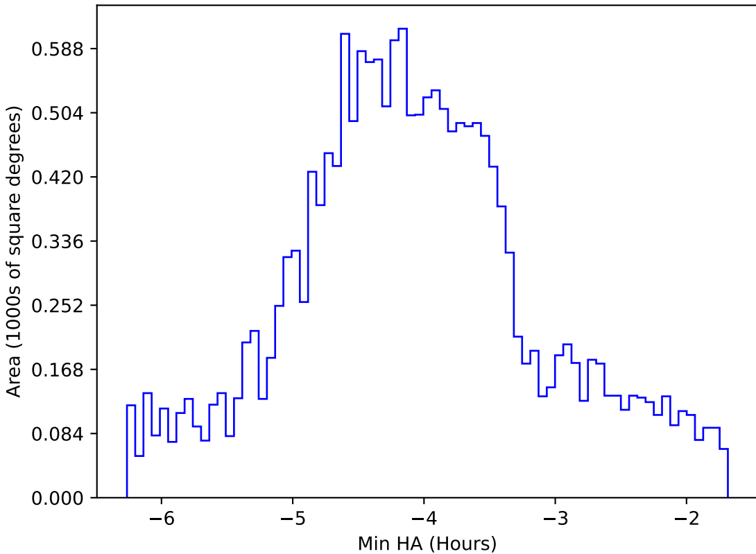
weather_cloudso0v3.5_10yrs WFD g band: Min HA
