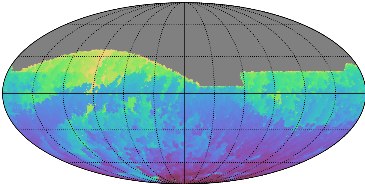
weather_cloudso0v3.5_10yrs All sky z band: Min HA
