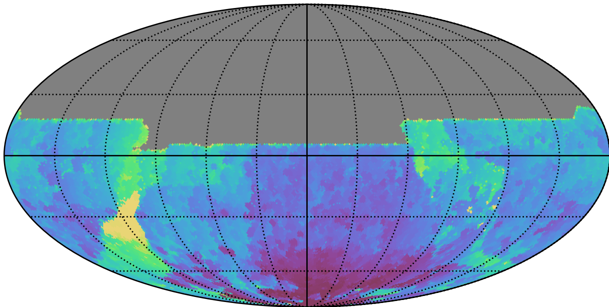
weather_cloudso0v3.5_10yrs All sky y band: Min HA
