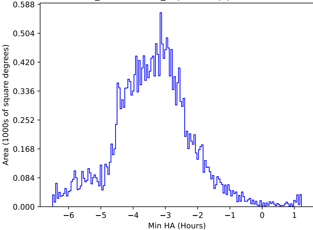
weather_cloudso0v3.5_10yrs All sky y band: Min HA
