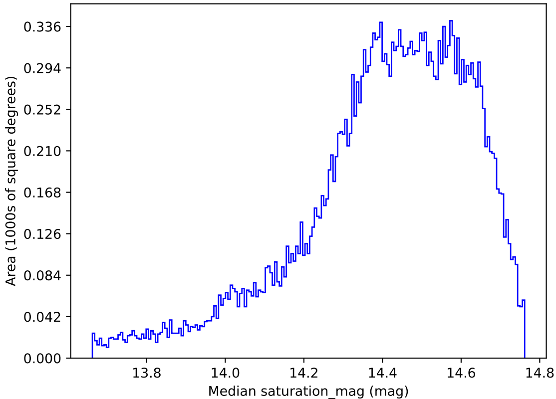
weather_cloudso0v3.5_10yrs All sky i band: Median saturation_mag
