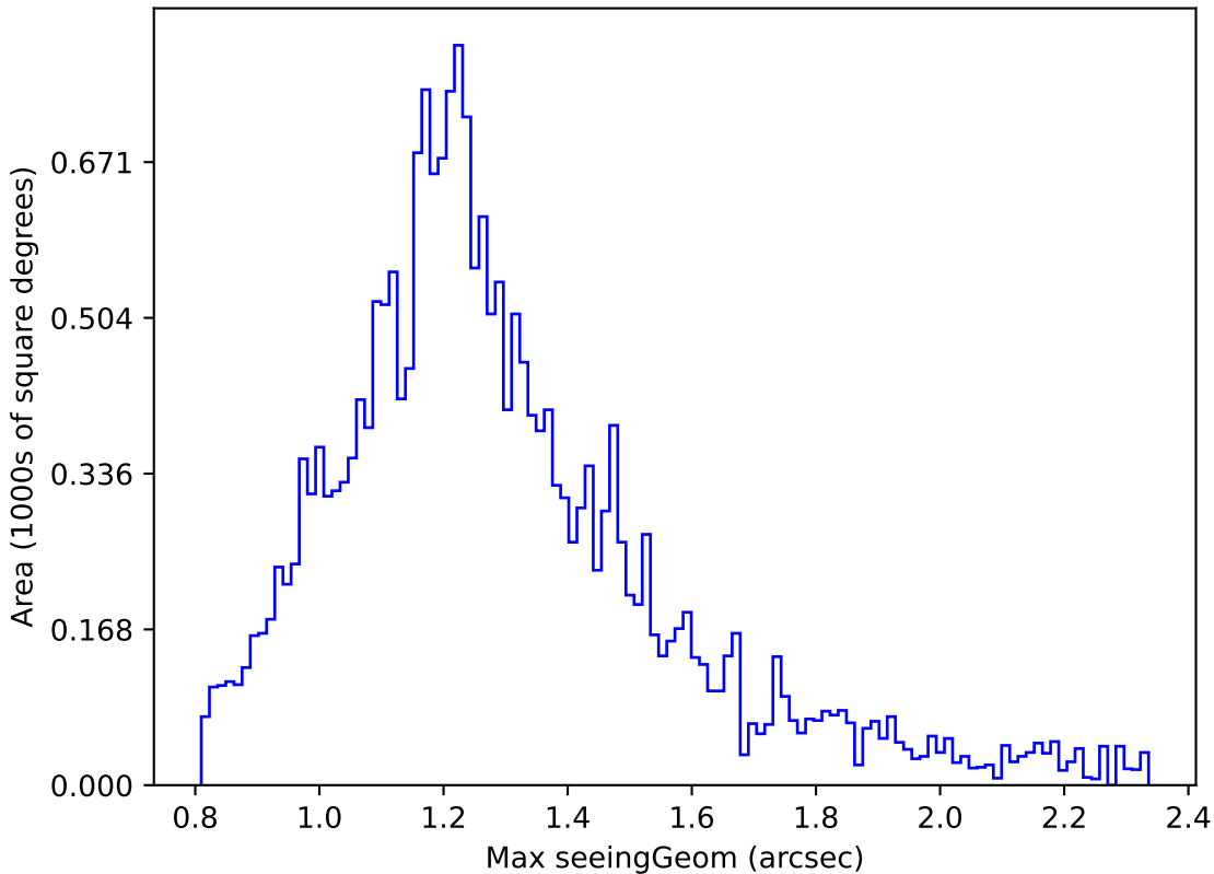
weather_cloudso0v3.5_10yrs Yr 1 y band: Max seeingGeom
