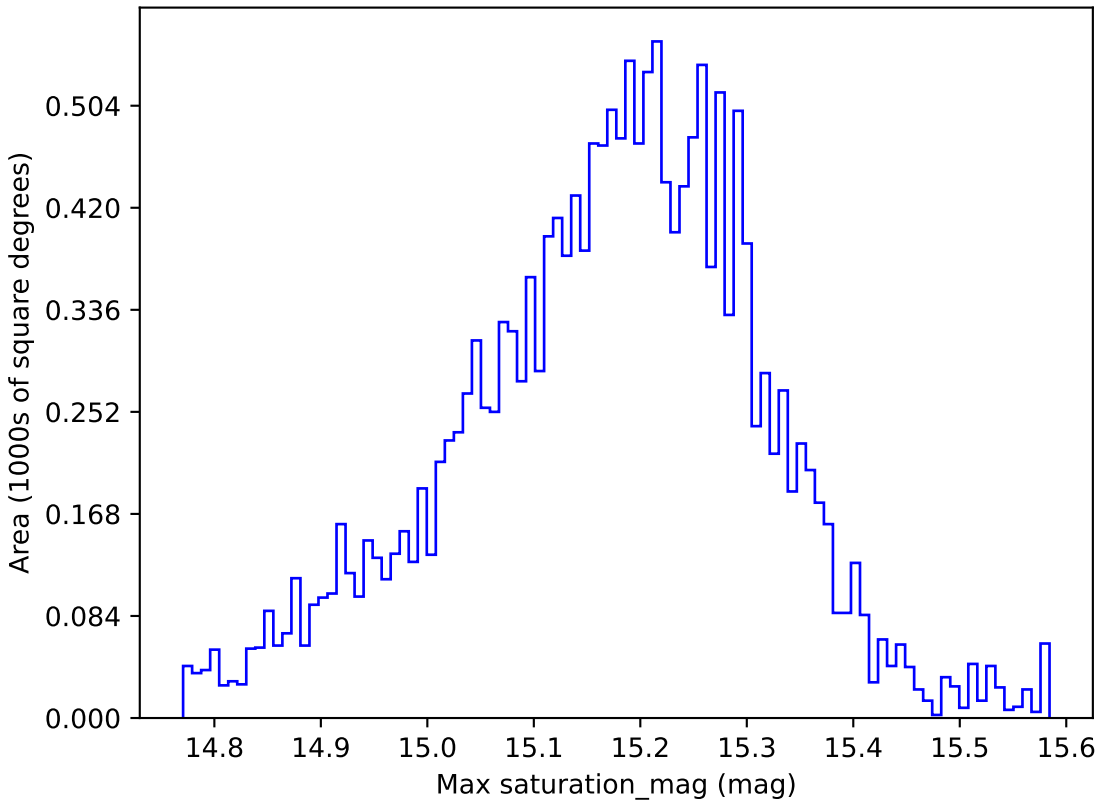
weather_cloudso0v3.5_10yrs WFD z band: Max saturation_mag
