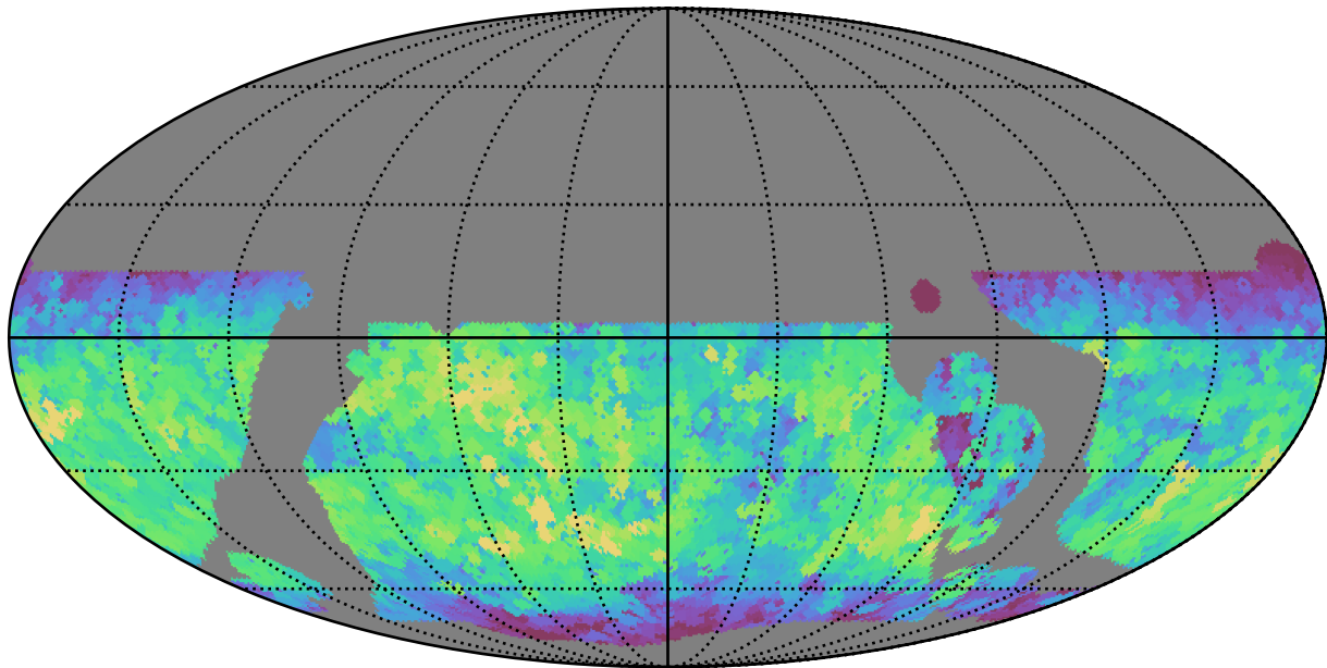
weather_cloudso0v3.5_10yrs WFD y band: Max saturation_mag
