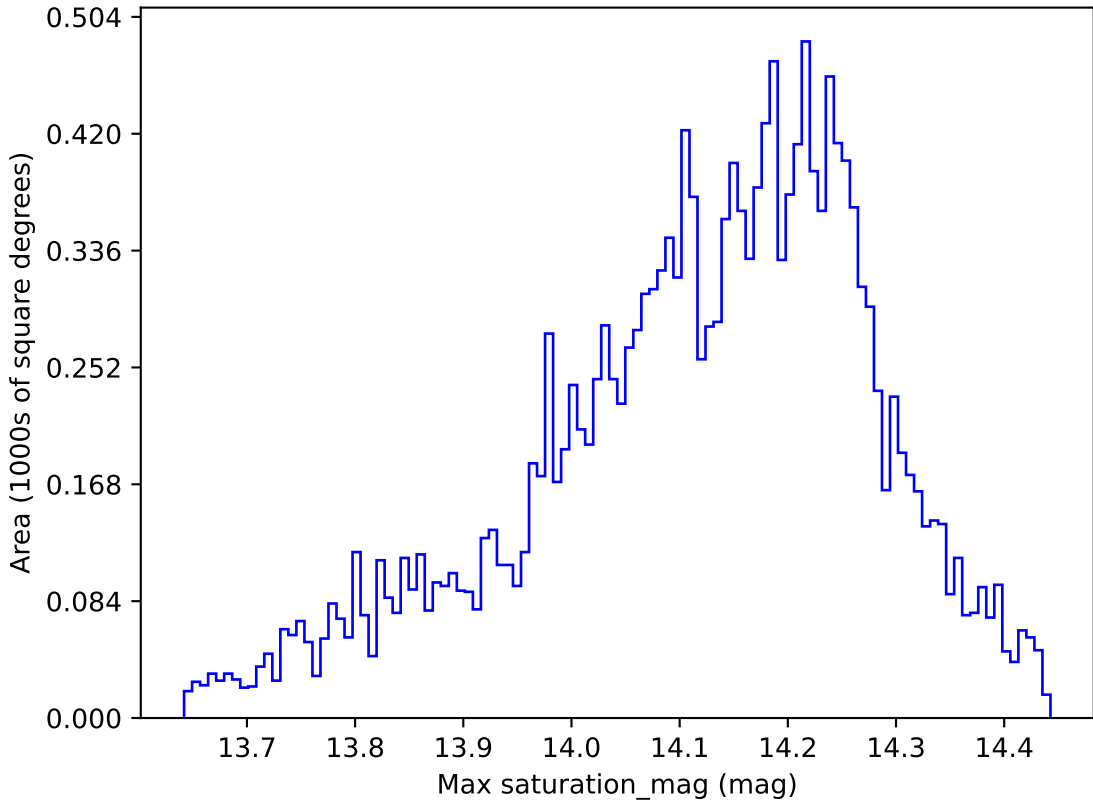
weather_cloudso0v3.5_10yrs WFD y band: Max saturation_mag
