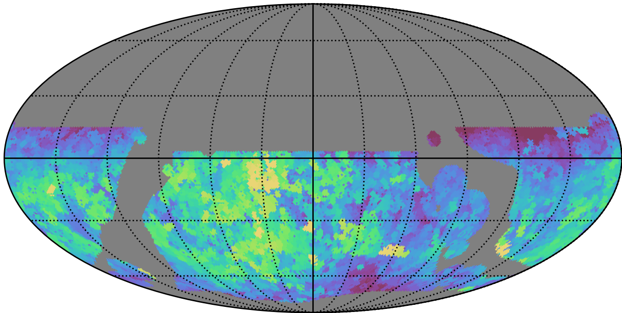
weather_cloudso0v3.5_10yrs WFD r band: Max saturation_mag
