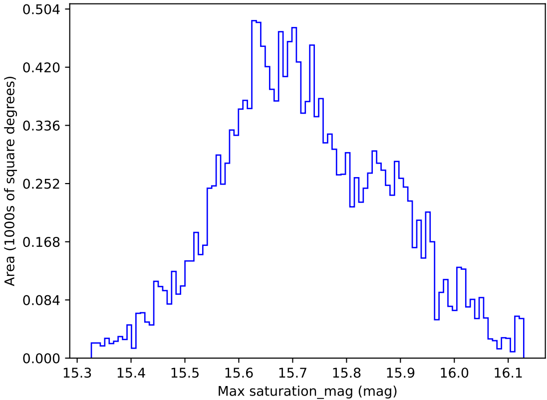
weather_cloudso0v3.5_10yrs WFD r band: Max saturation_mag
