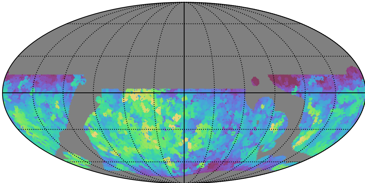
weather_cloudso0v3.5_10yrs WFD i band: Max saturation_mag
