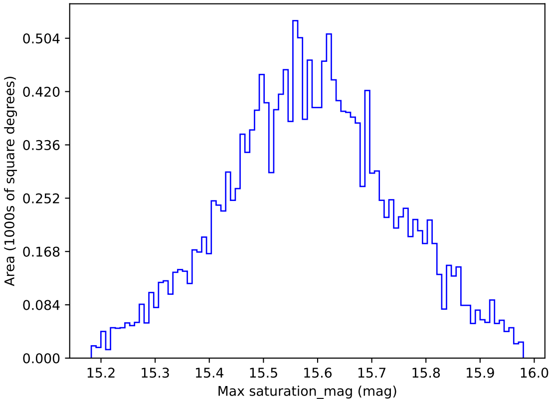
weather_cloudso0v3.5_10yrs WFD i band: Max saturation_mag
