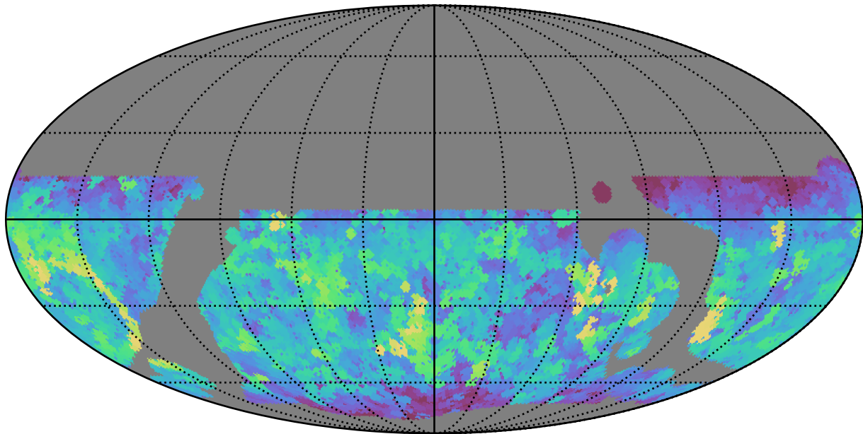
weather_cloudso0v3.5_10yrs WFD g band: Max saturation_mag
