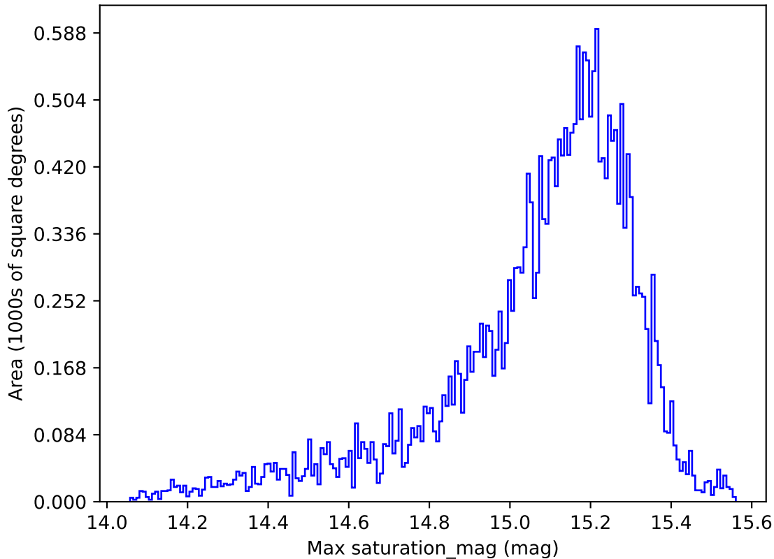
weather_cloudso0v3.5_10yrs All sky z band: Max saturation_mag
