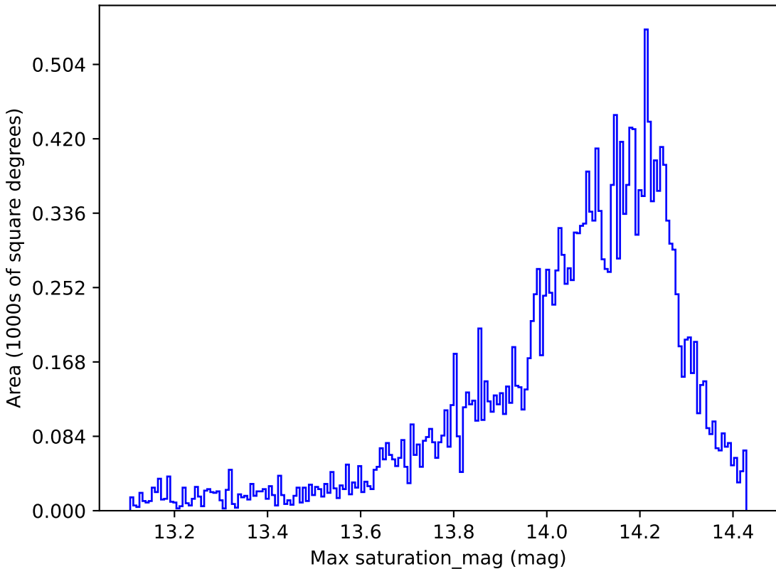
weather_cloudso0v3.5_10yrs All sky y band: Max saturation_mag
