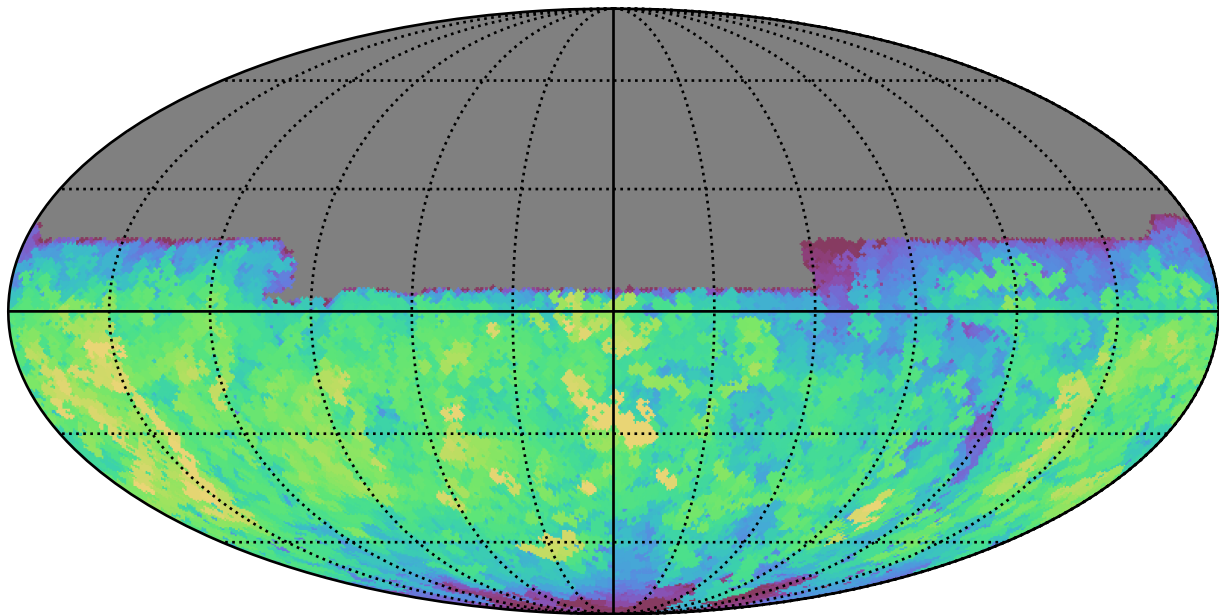
weather_cloudso0v3.5_10yrs All sky u band: Max saturation_mag
