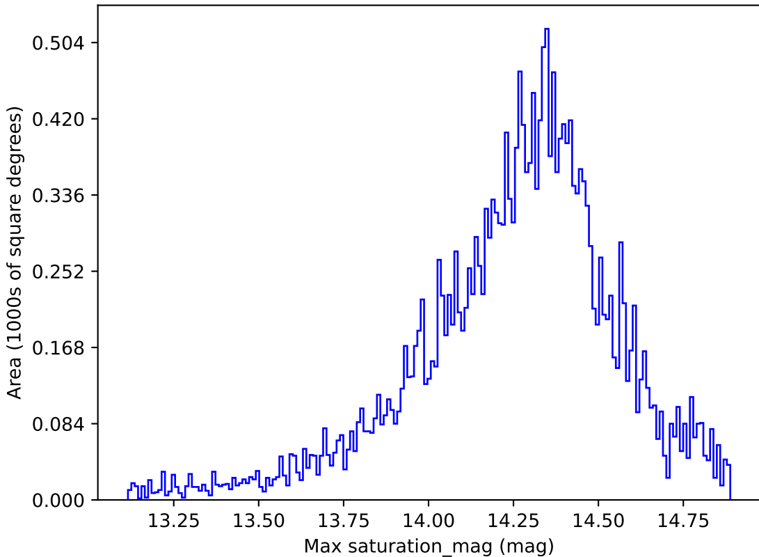
weather_cloudso0v3.5_10yrs All sky u band: Max saturation_mag
