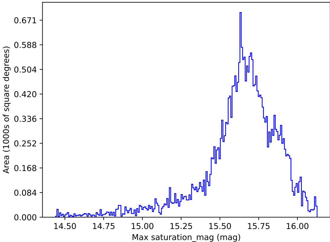
weather_cloudso0v3.5_10yrs All sky r band: Max saturation_mag
