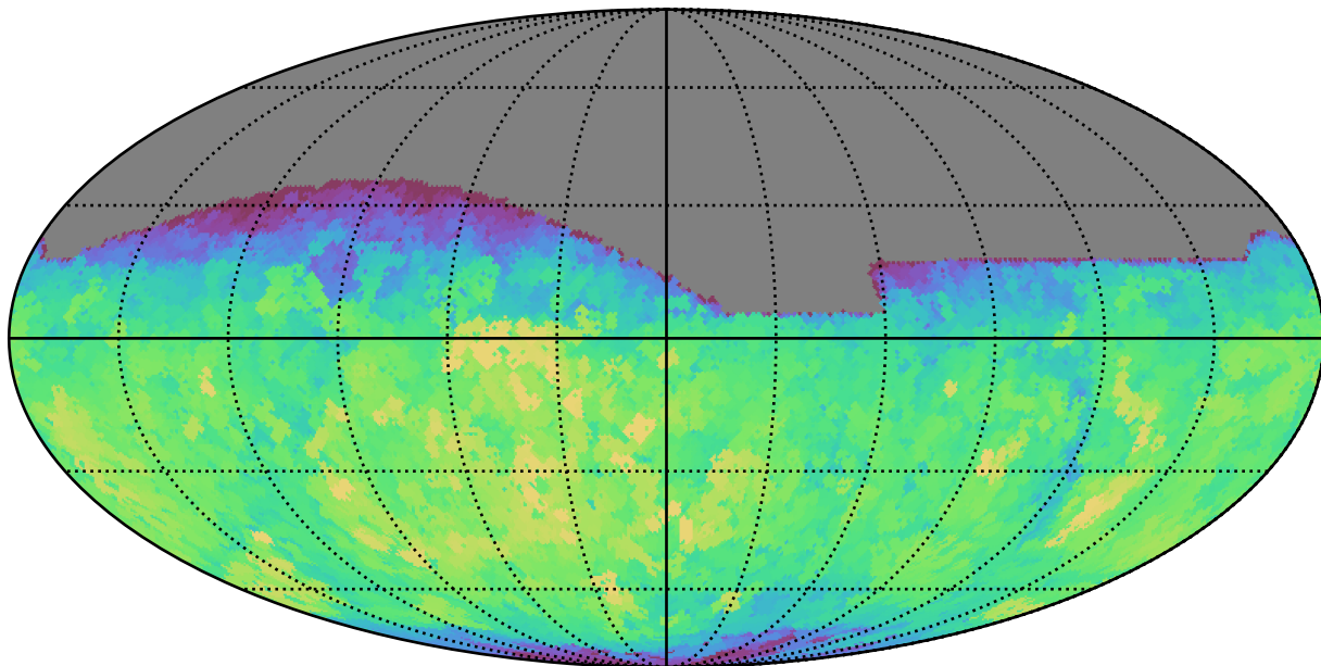
weather_cloudso0v3.5_10yrs All sky i band: Max saturation_mag
