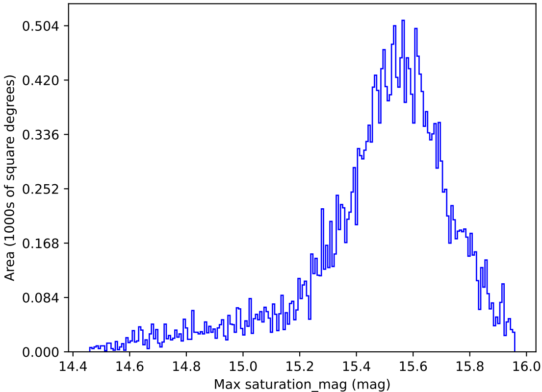
weather_cloudso0v3.5_10yrs All sky i band: Max saturation_mag
