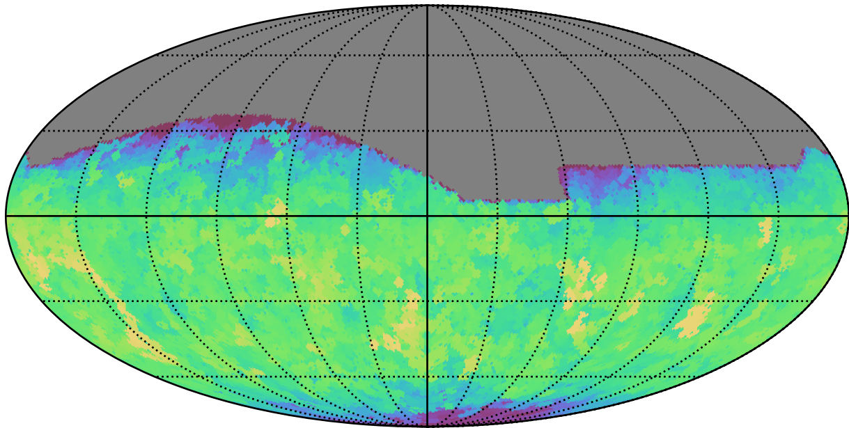
weather_cloudso0v3.5_10yrs All sky g band: Max saturation_mag
