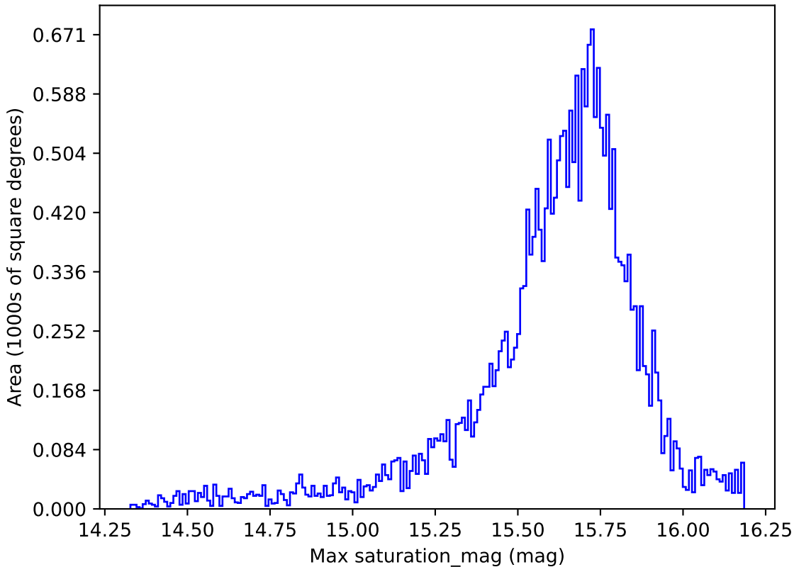
weather_cloudso0v3.5_10yrs All sky g band: Max saturation_mag
