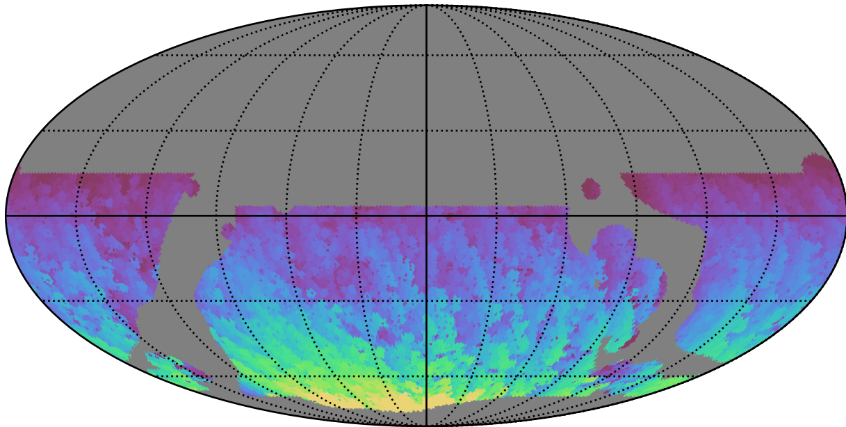
weather_cloudso0v3.5_10yrs WFD y band: Max HA
