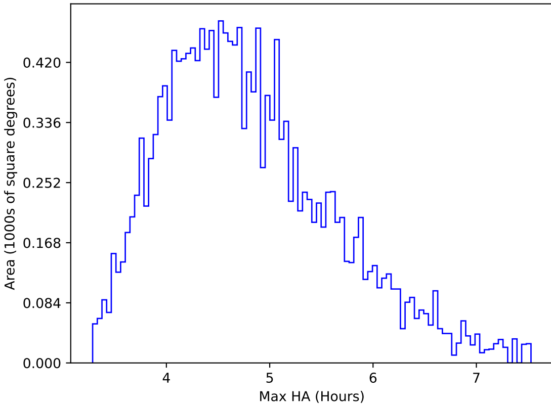
weather_cloudso0v3.5_10yrs WFD y band: Max HA
