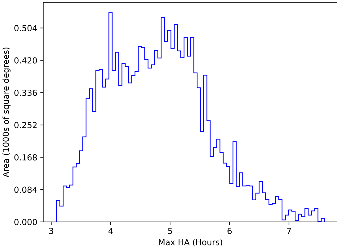
weather_cloudso0v3.5_10yrs WFD i band: Max HA
