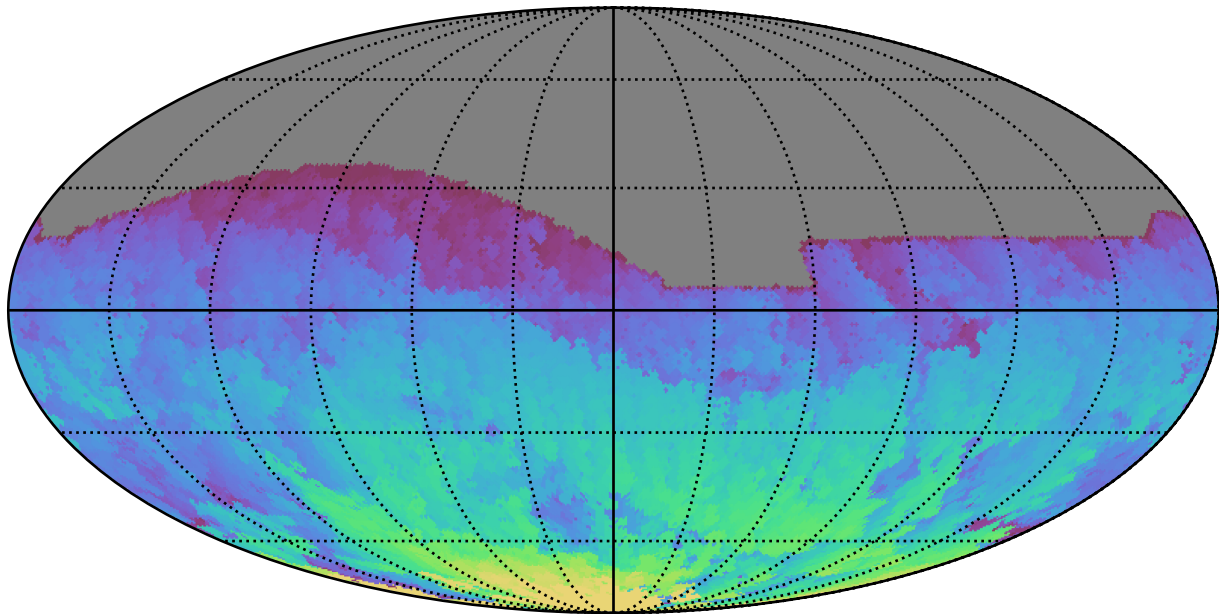
weather_cloudso0v3.5_10yrs All sky i band: Max HA
