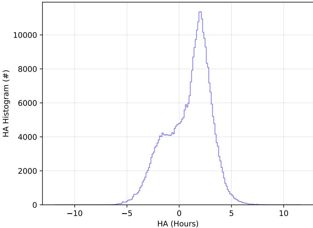
weather_cloudso0v3.5_10yrs WFD y band: HA Histogram
