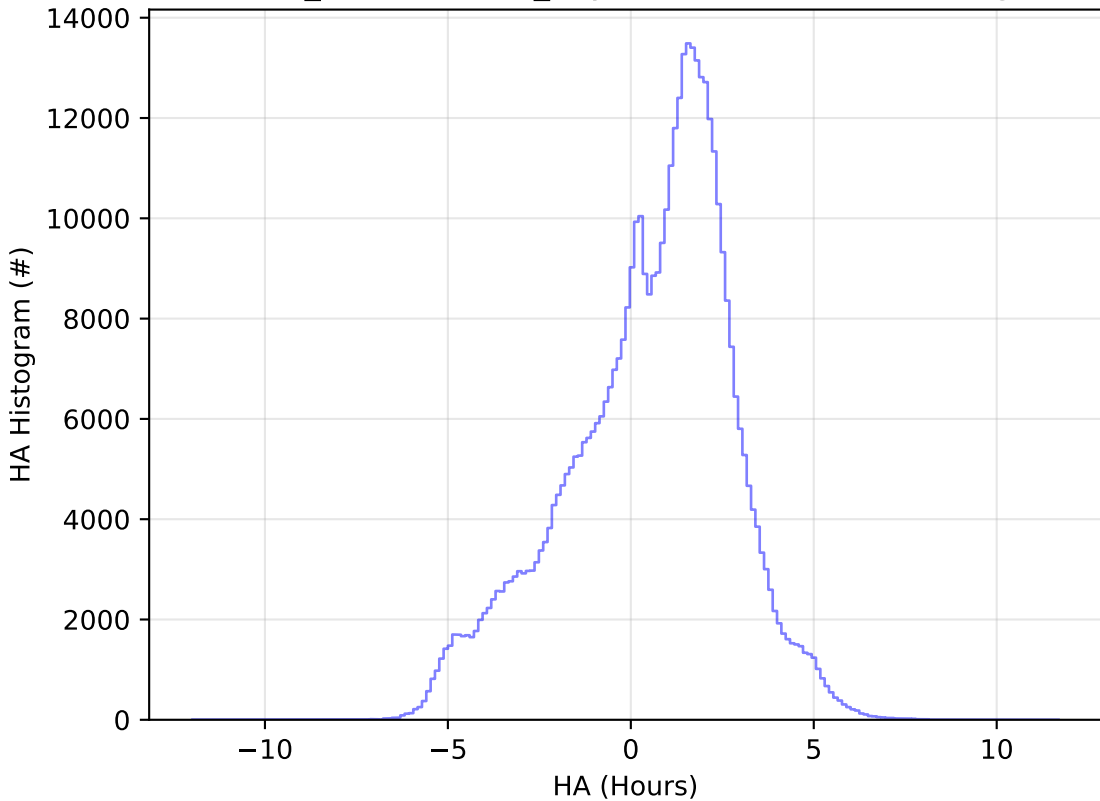
weather_cloudso0v3.5_10yrs WFD i band: HA Histogram
