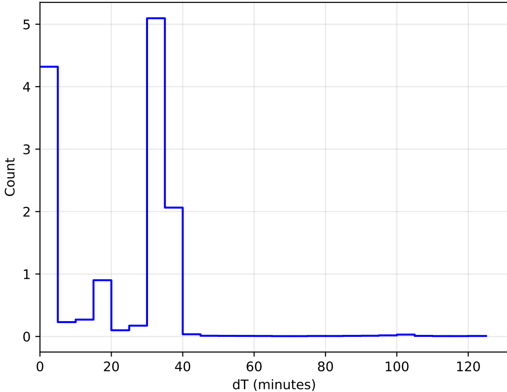
weather_cloudso0v3.5_10yrs All sky: DeltaT Histogram
