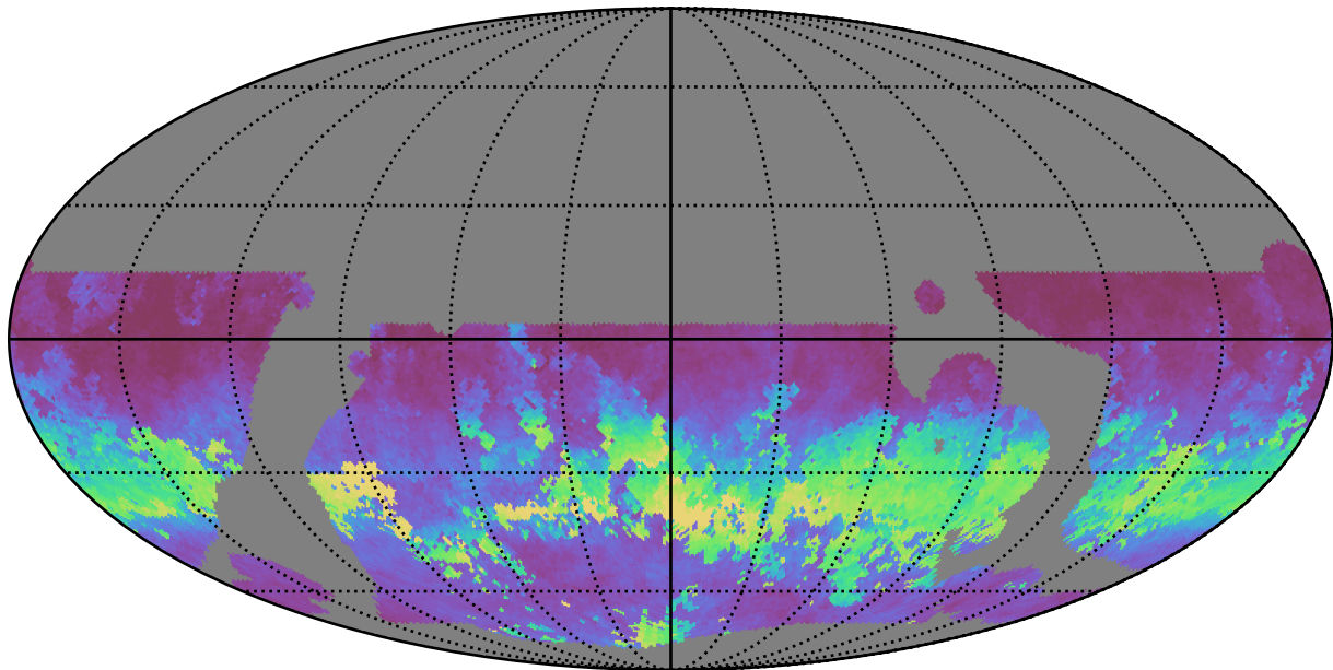
weather_cloudso0v3.5_10yrs WFD i band: AngleRms rotSkyPos
