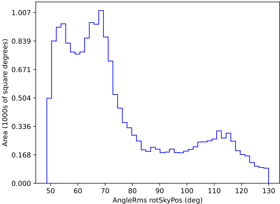
weather_cloudso0v3.5_10yrs WFD i band: AngleRms rotSkyPos
