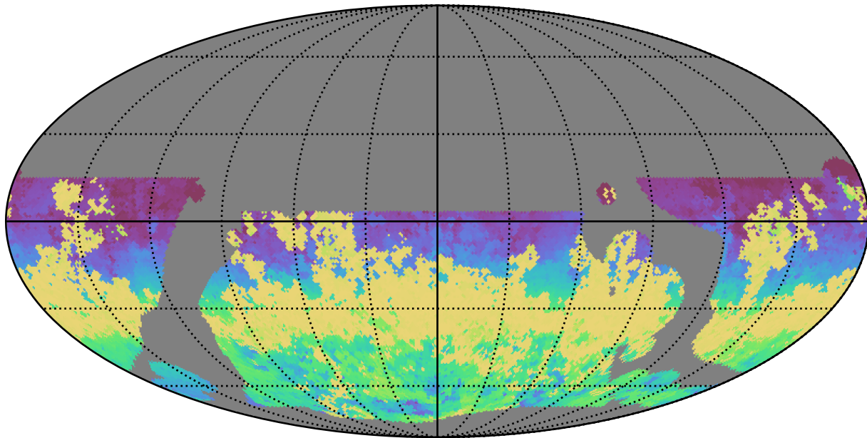
weather_cloudso0v3.5_10yrs WFD z band: AngleRange rotSkyPos
