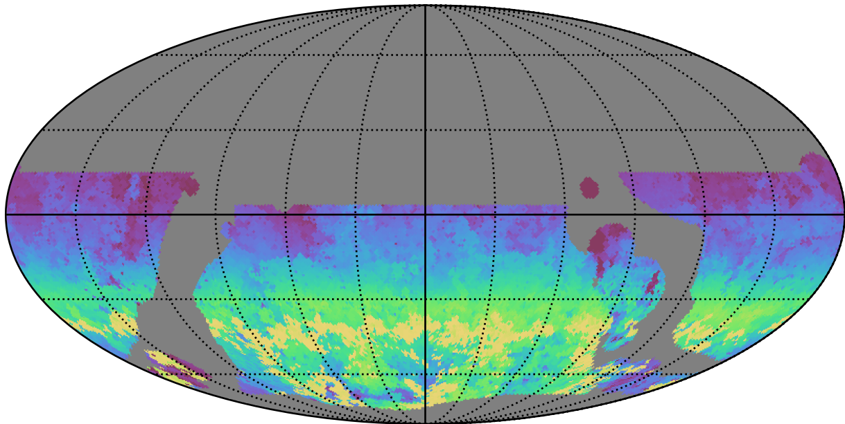
weather_cloudso0v3.5_10yrs WFD y band: AngleRange rotSkyPos
