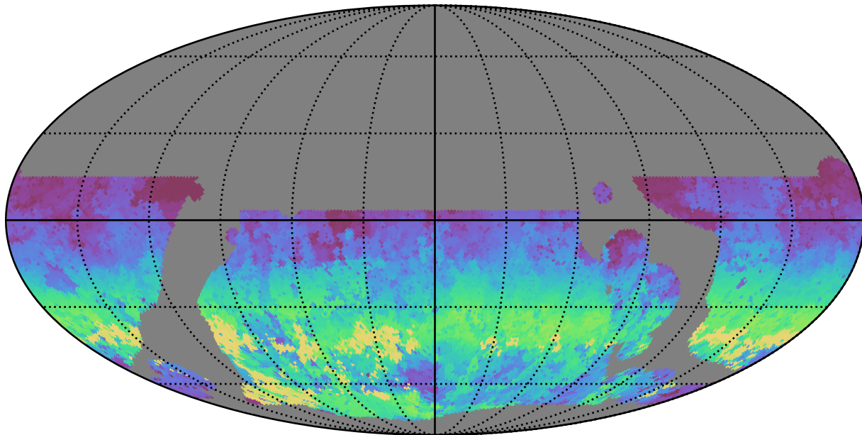
weather_cloudso0v3.5_10yrs WFD u band: AngleRange rotSkyPos
