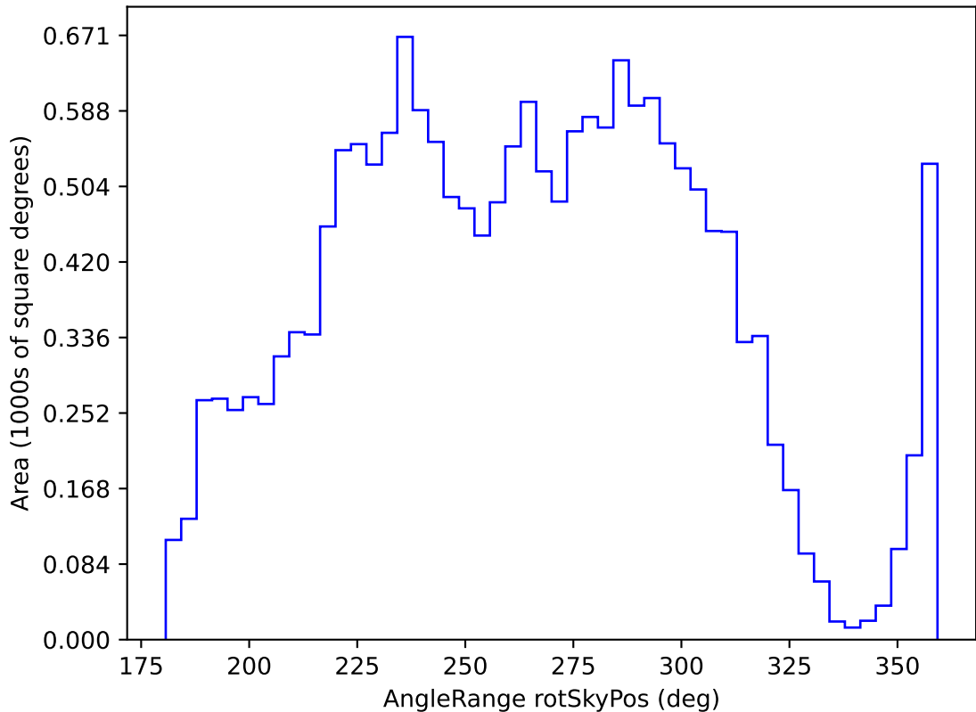
weather_cloudso0v3.5_10yrs WFD u band: AngleRange rotSkyPos
